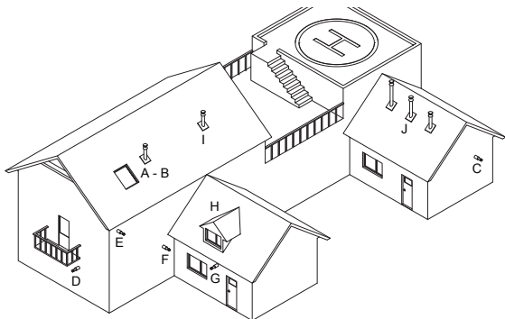
Rys. 7. Możliwe warianty wyprowadzenia koncentrycznego systemu powietrzno- spalinyowego dla urządzeń z serii LEO
