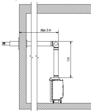
Rys. 8. Sposób wyprowadzenia koncentrycznego systemu kominowego przez ścianę
