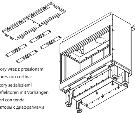
Figur 14. LEO70 serien - deflectors med membraner
