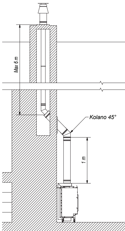
Rys. 10. Sposób instalacji urządzenia z użyciem istniejącego komina
