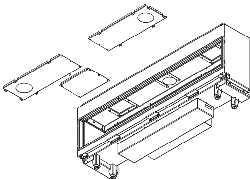
Rys. 13. Demontaż deflektorów LEO100 i LEO200
